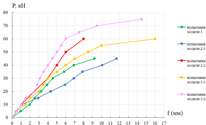
Рис. 4. Графики перемещений верха моделей 1, 2-1, 2-2, 3-1, 3-2
