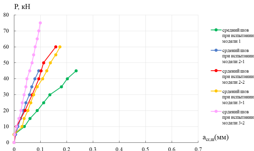
Рис. 5. Графики ширины раскрытия межблочных строительных швов (средний шов) при испытании моделей 1, 2-1, 2-2, 3-1, 3-2
