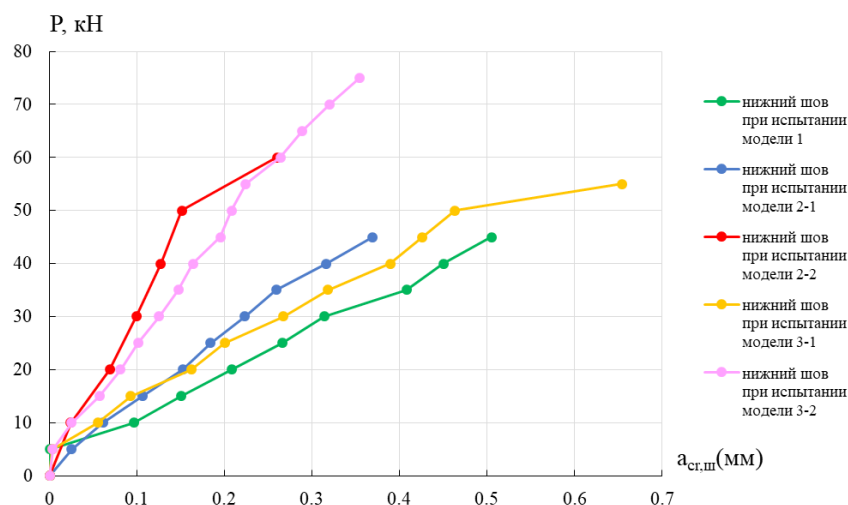
Рис. 6. Графики ширины раскрытия межблочных строительных швов (нижний шов) при испытании моделей 1, 2-1, 2-2, 3-1, 3-2
