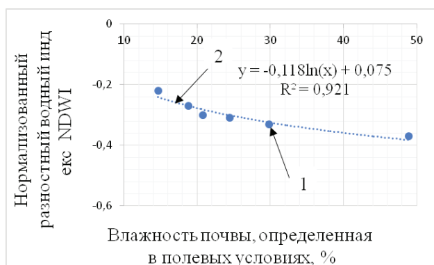
Рис. 3. Связь влажности почвы, определенная в полевых условиях, с нормализованным разностным водным индексом NDWI:
