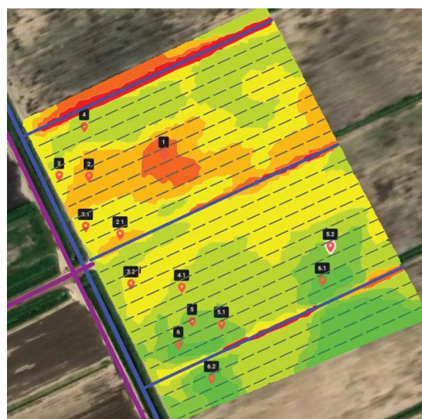
Рис. 2. Оперативная карта влажности, полученная в результате расчета нормализованного водного индекса NDWI
