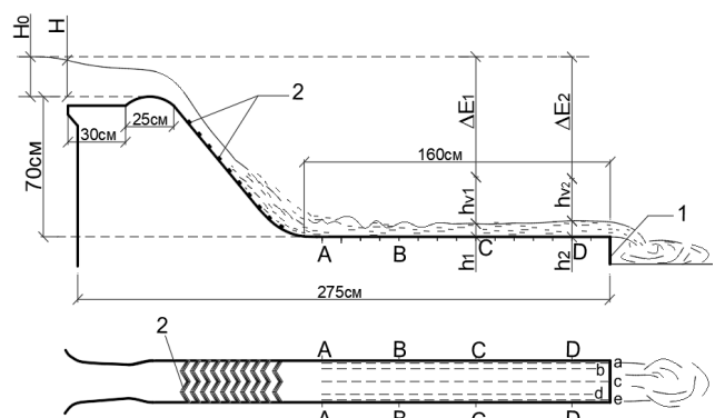
Рис. 1. Принципиальная схема модели водосливной плотины:
