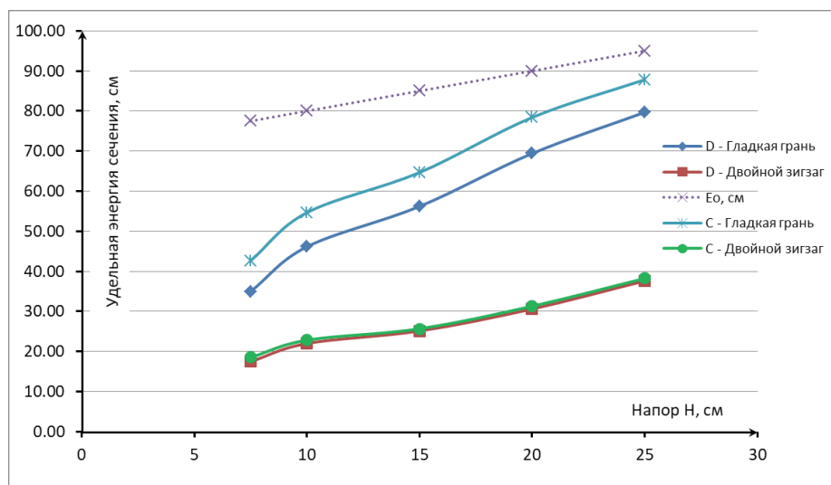
Рис. 3. Кривые изменения удельной энергии в поперечных створах С и Д
