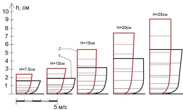
Рис. 4. Эпюры скорости в центральном продольном створе «С» и поперечном створе «Д»:
